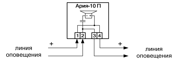
Рис.1. Схема подключения.
