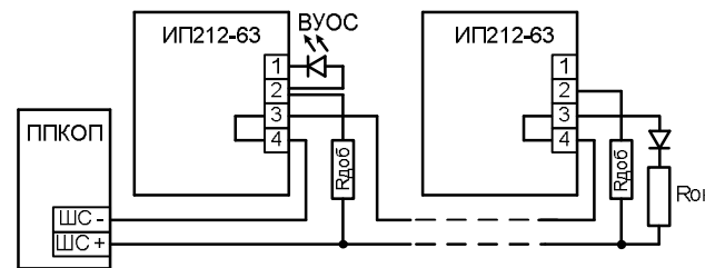
Рис.2 Типовая схема включения извещателя для приборов с переполюсовкой шлейфа сигнализации. Величина резисторов R_{ок} и R_{добр} определяется в соответствии с техническим описанием ППКОП
