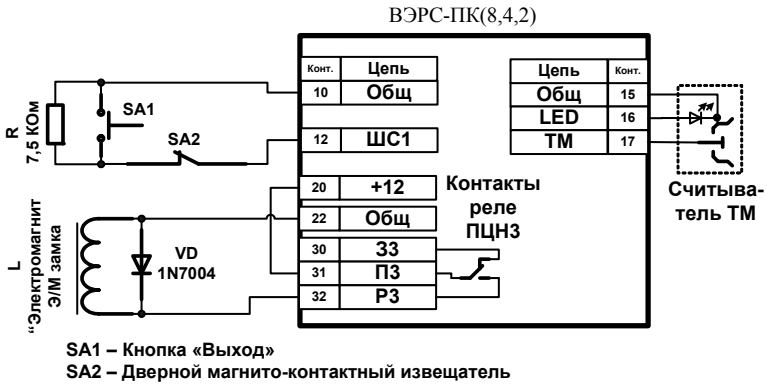
Рисунок Б5. Схема организации Точки доступа.
