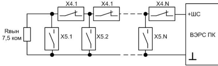
Рисунок Б10. Схема включения охранных извещателей в ЩСО.
