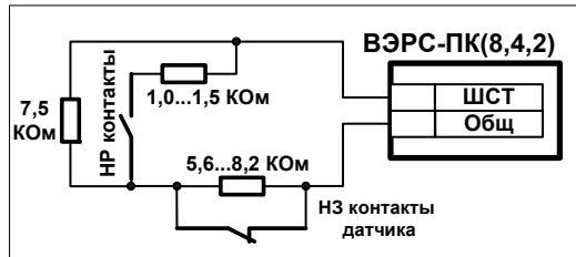
Рисунок Б11. Схема включения технологических датчиков в ЩСТ.
