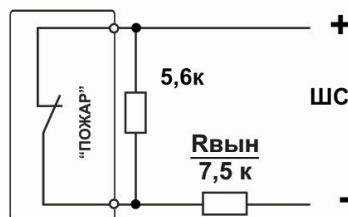
Рис. 7. Организация двухпорогового шлейфа пожарной сигнализации
