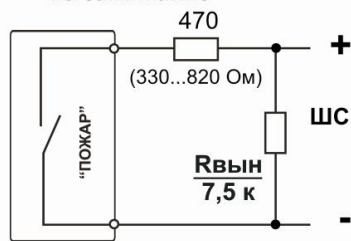
Рис. 7. Организация двухпорогового шлейфа пожарной сигнализации
